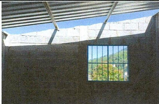
Foto 6: Sustrucción cubierta de techo a lámina troquelada calibre 26 e instalación de estructura metálica
